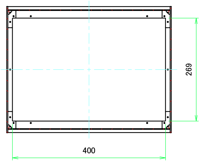
B-B ( 1 : 6 )
