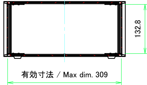
A-A ( 1 : 6 )
