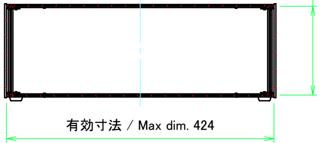
C-C ( 1 : 6 )
